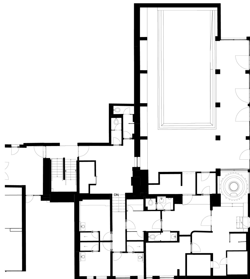
Erdgeschoss- Spa 1 : 100
